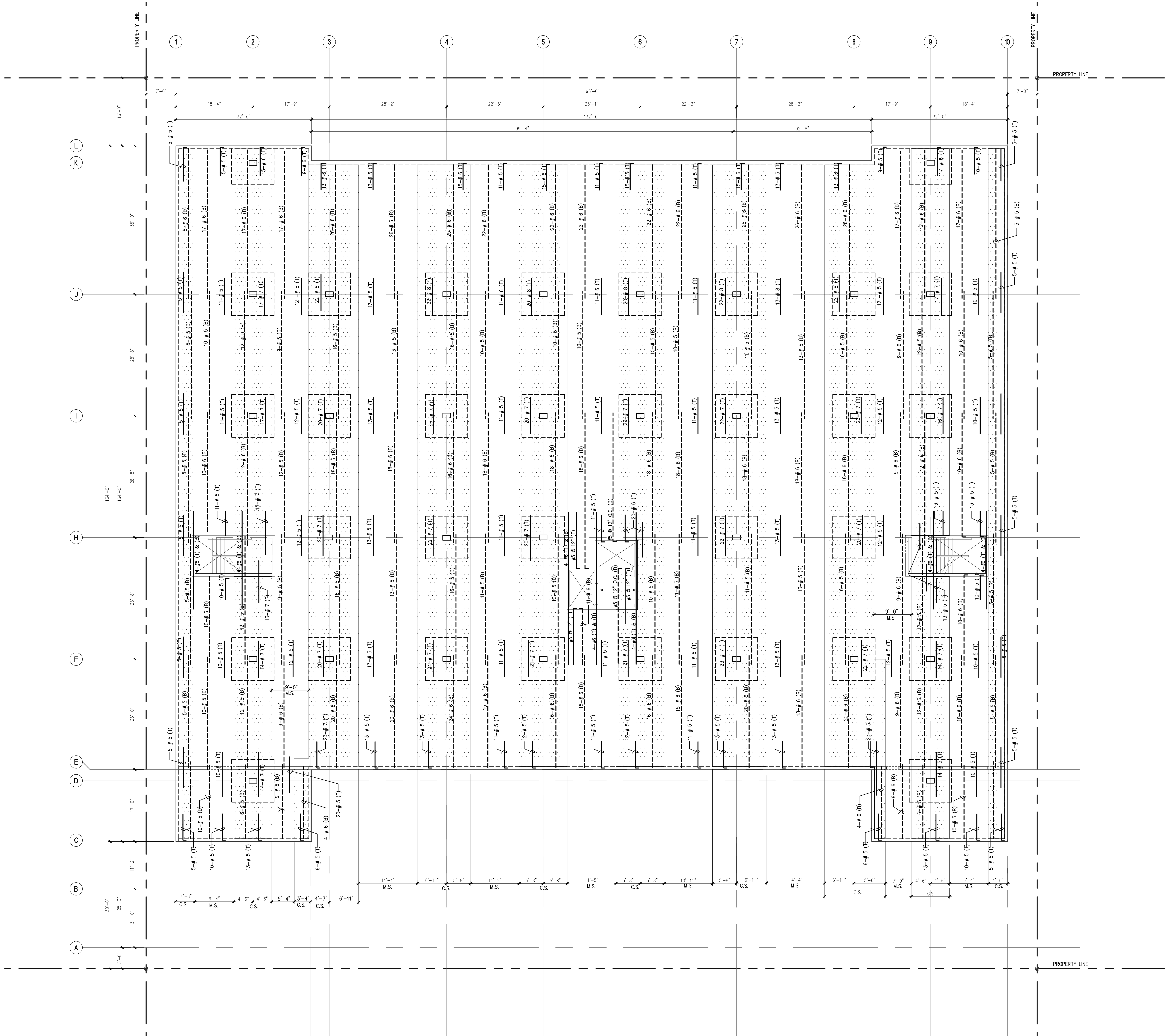
PODIUM PLAN SCALE: 1/8" = 1'-0"
